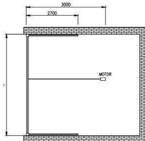
차고문 평면도
