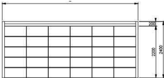
입면도
