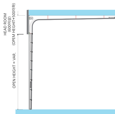
HI-LIFT TYPE
