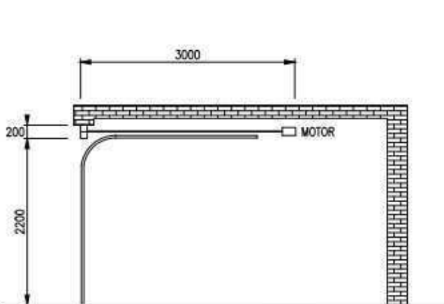
차고문 측면도
